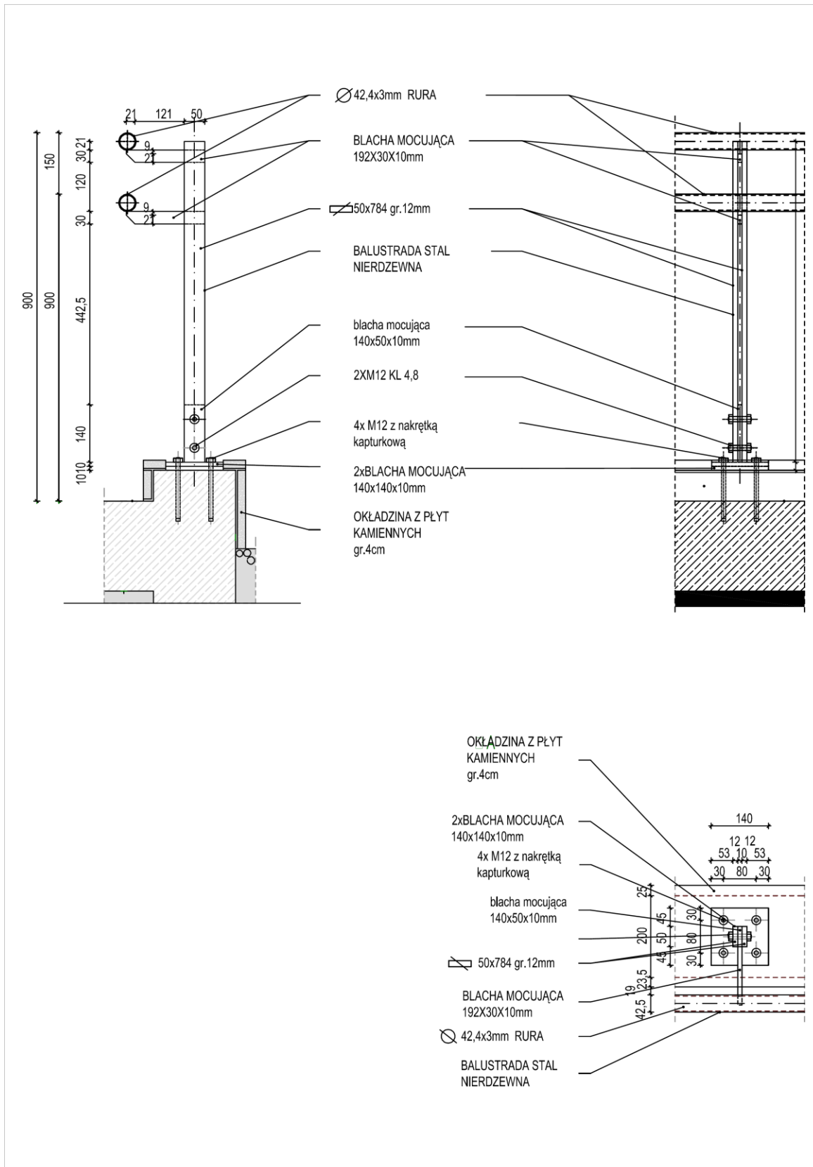
Rysunek montażu balustrady
