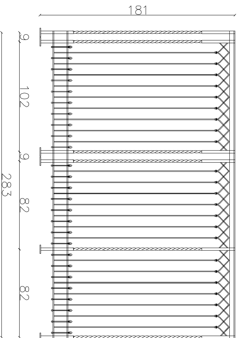
Widok ogrodzenia skala 1:5
