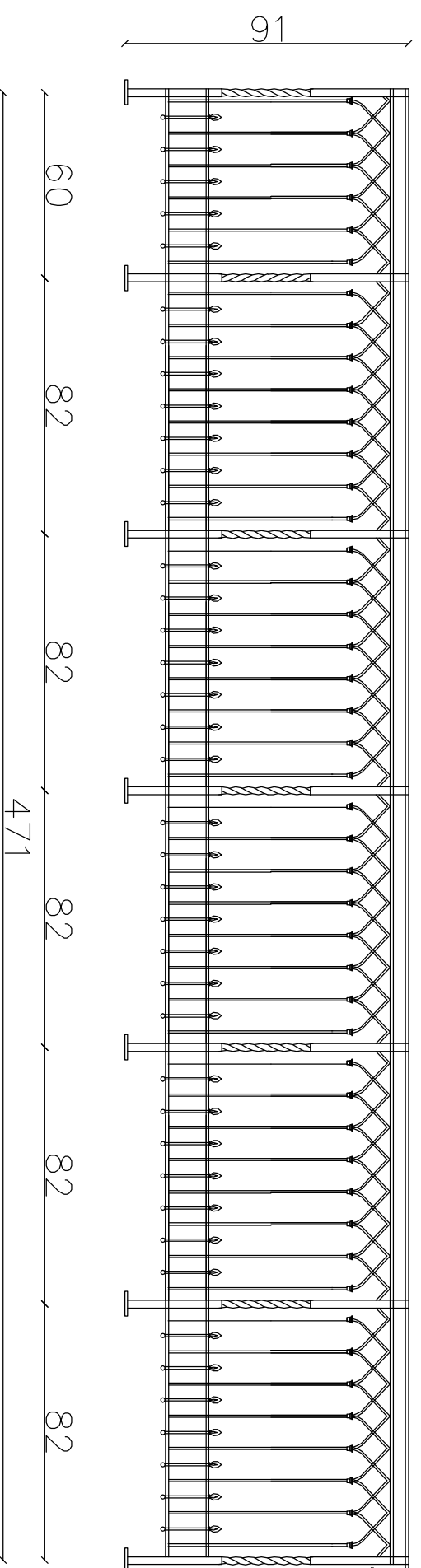
Widok balustrady skala 1:5
