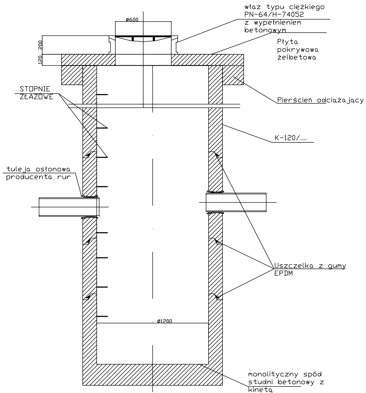
STUDZIENKA KANALIZACYJNA REWIZYJNA
