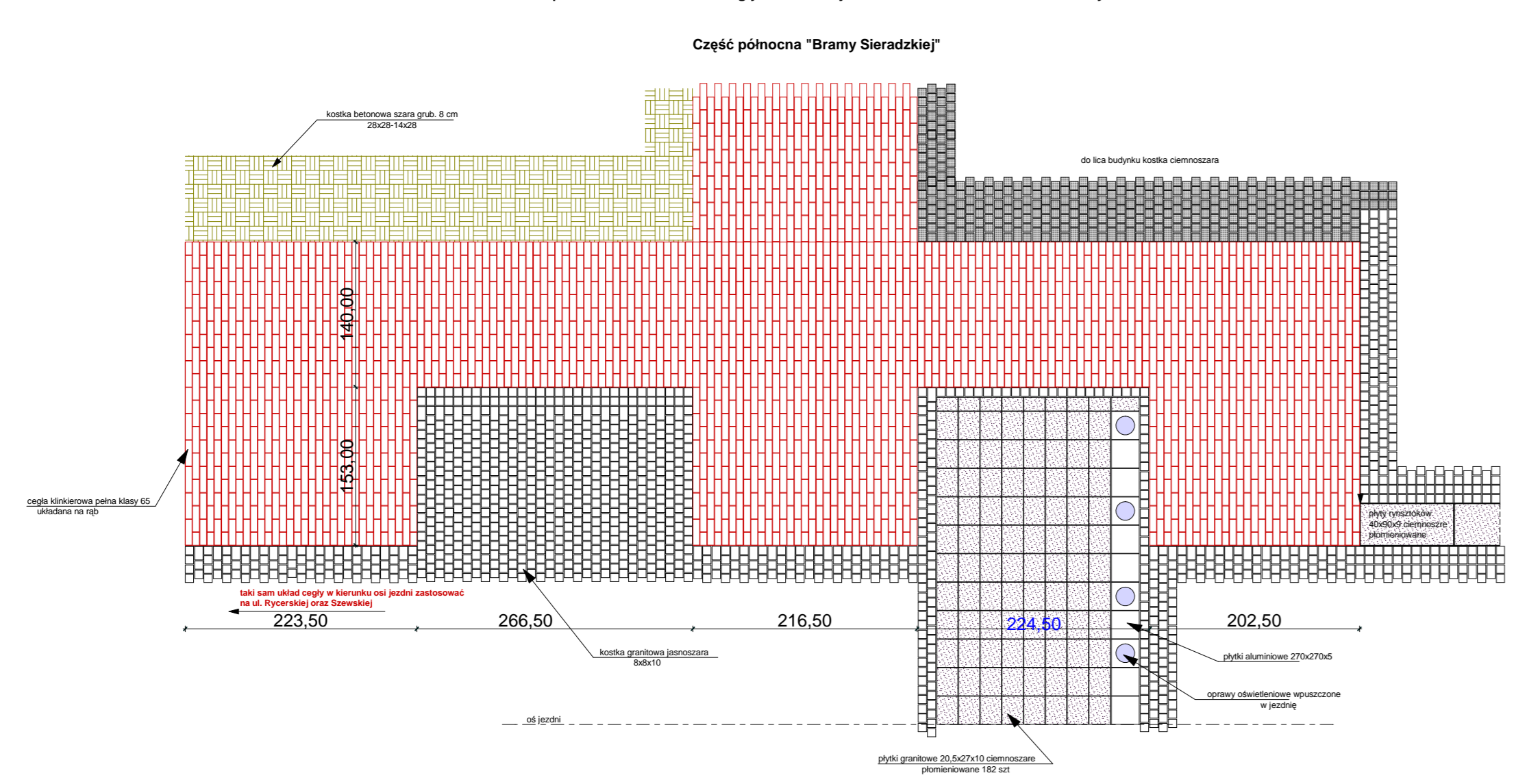
Sposób układania kostki i cegły klinkowej w elementach ścian murów ochronnych
