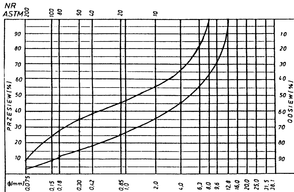
asfaltowego dla KR 1-2 Rys. 10. Krzywe graniczne uziarnienia mieszanki mineralnej 0+12,8 mm do warstwy wiążącej, wyrównawczej i wzmacniającej z betonu asfaltowego dla KR 1-2
