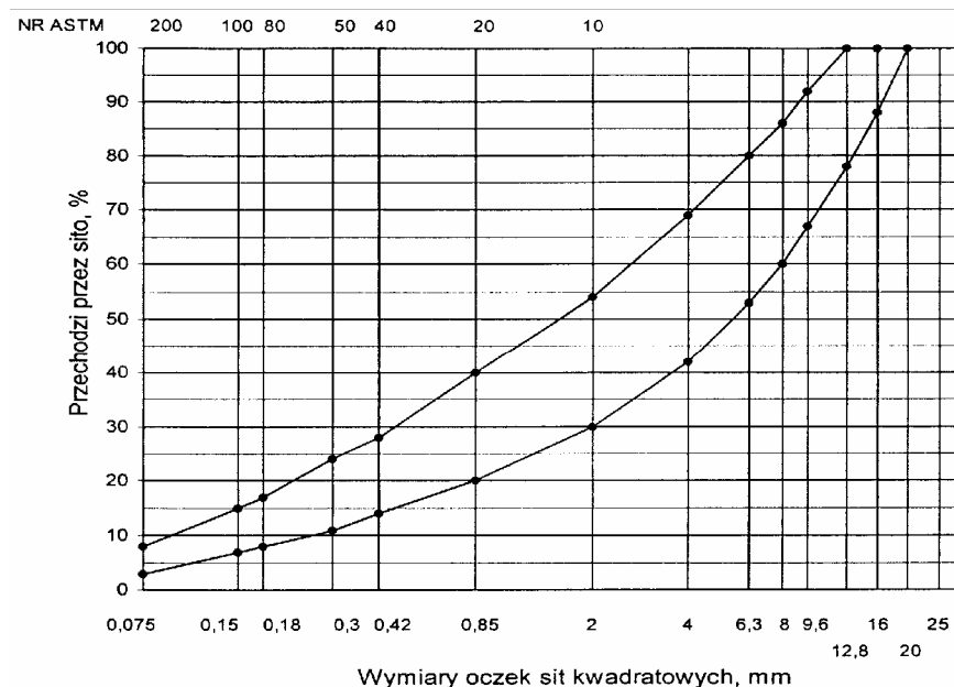
Rys. 1. Krzywe graniczne uziarnienia mieszanki mineralnej BA od 0 do 16 mm do warstwy wiążącej, wyrównawczej nawierzchni drogi o obciążeniu ruchem KR1 lub KR2
