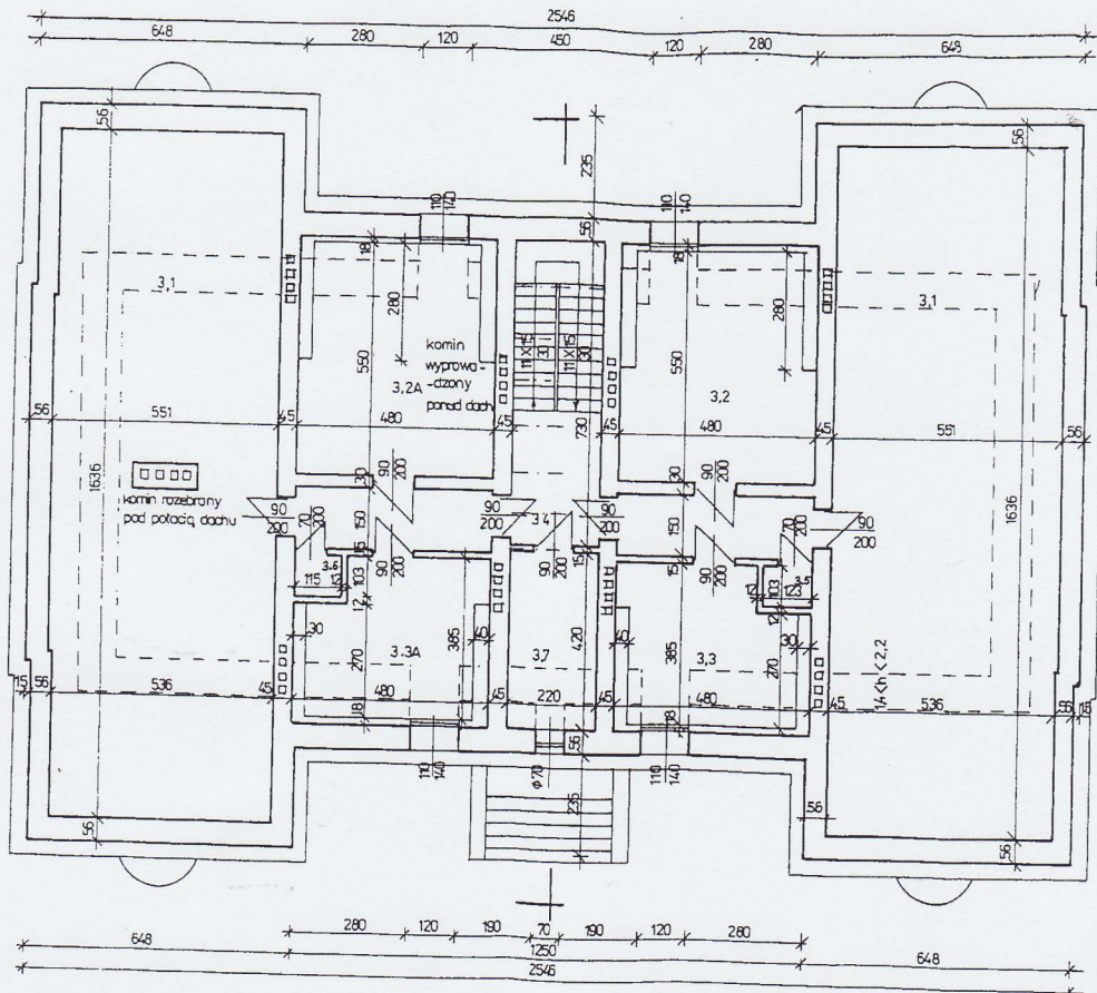
RZUT PODDASZA
